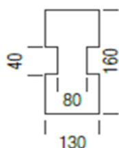
DIMENSIONE PALO
